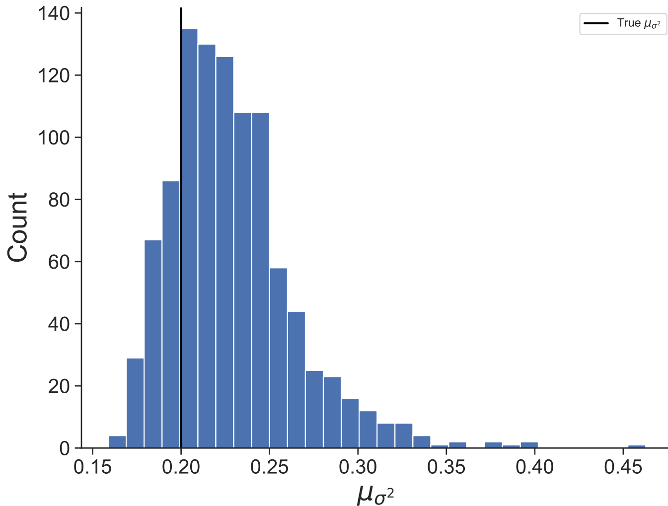
Dataset 18
