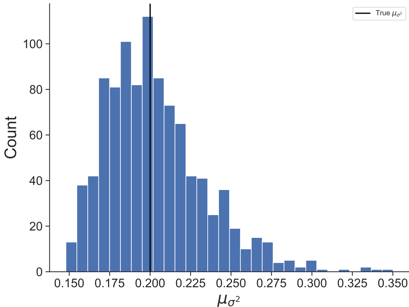
Dataset 40
