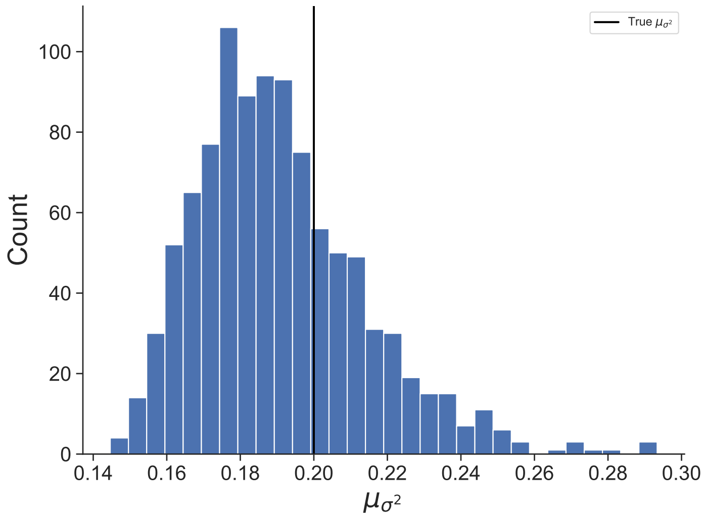
Dataset 34
