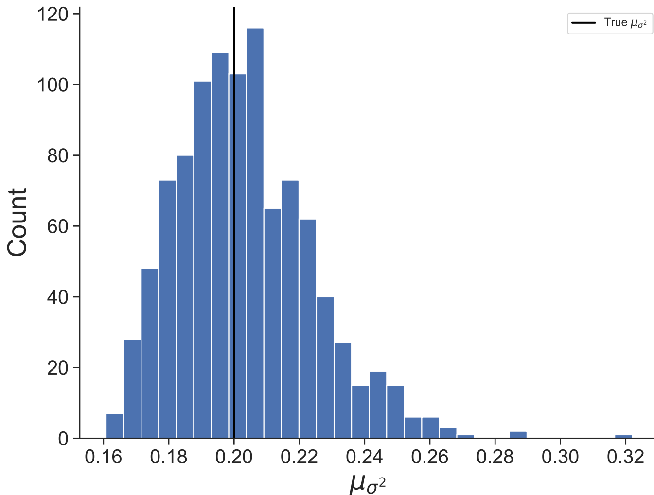
Dataset 27
