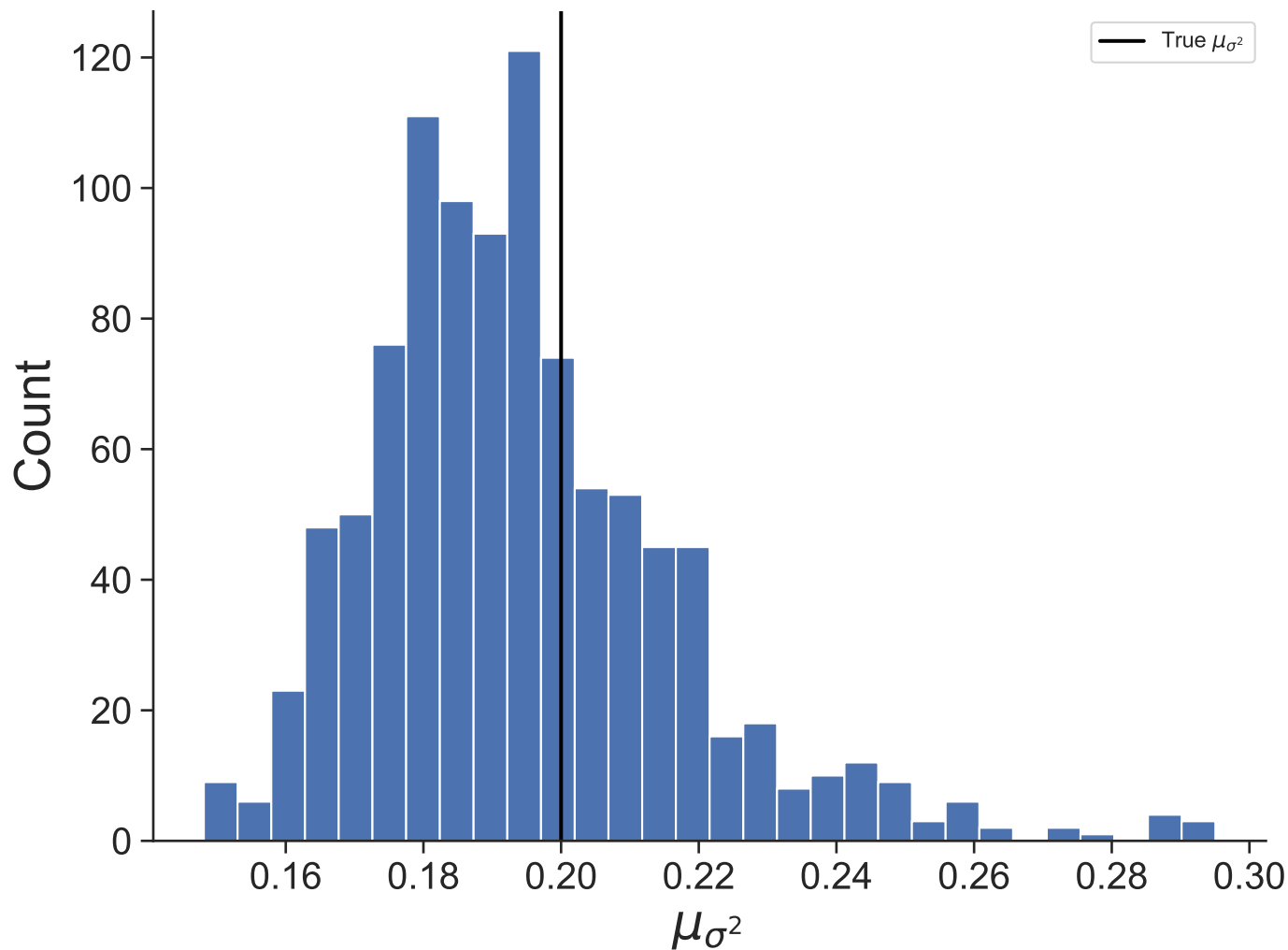
Dataset 30
