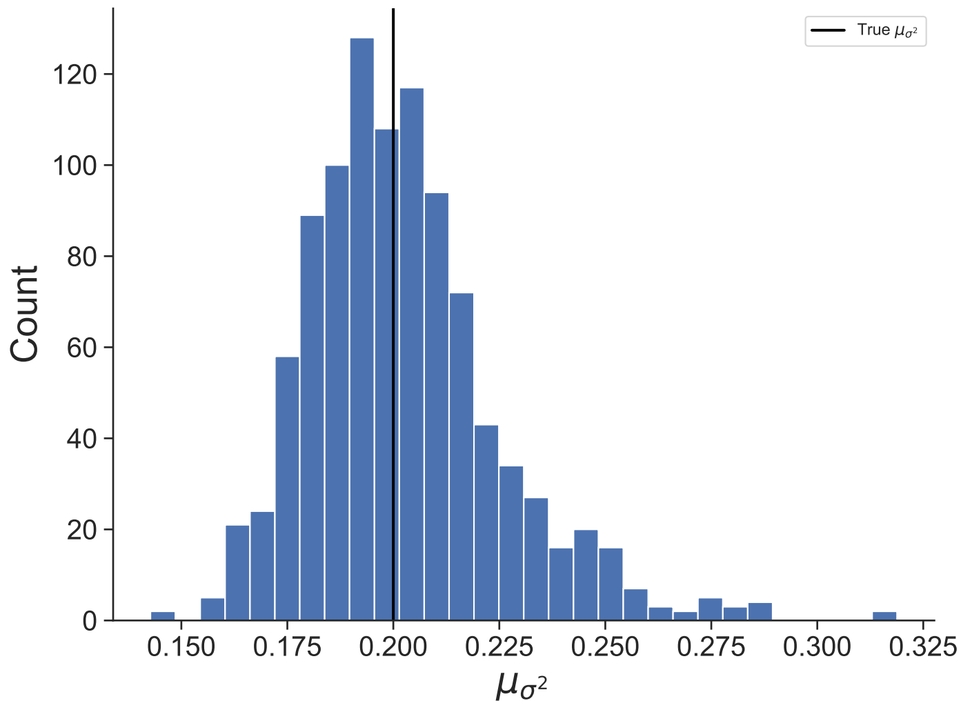
Dataset 25
