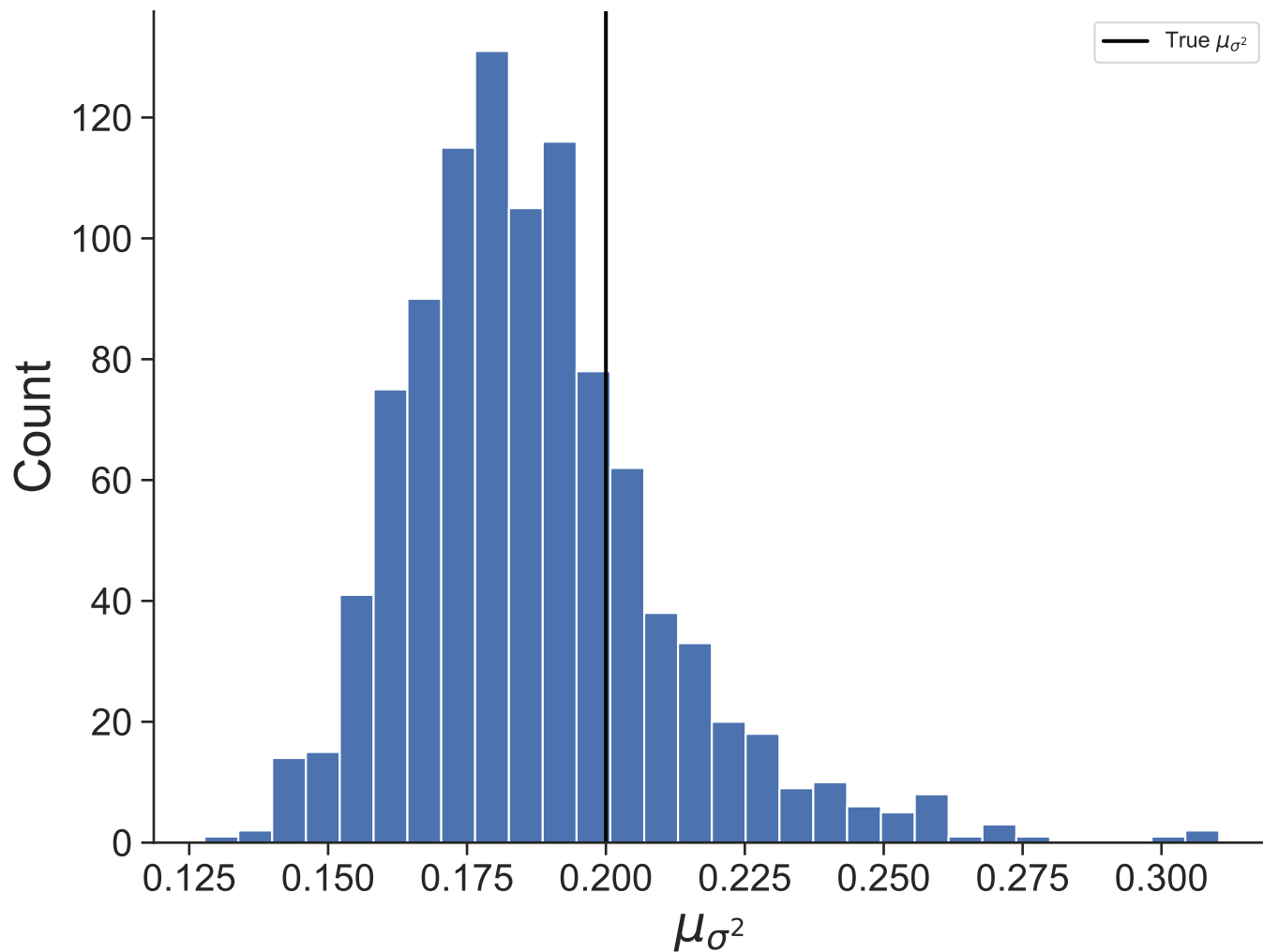
Dataset 1
