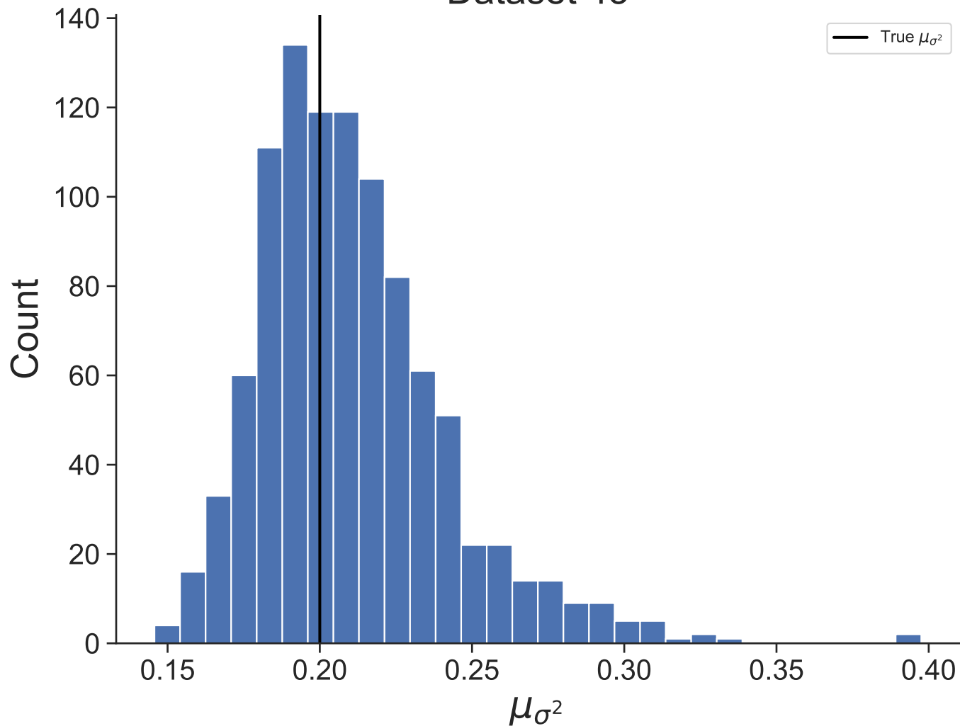
Dataset 43
