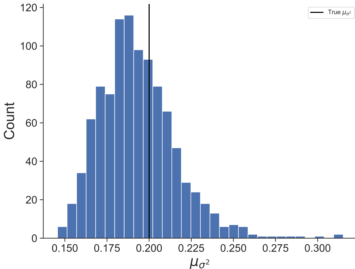
Dataset 32
