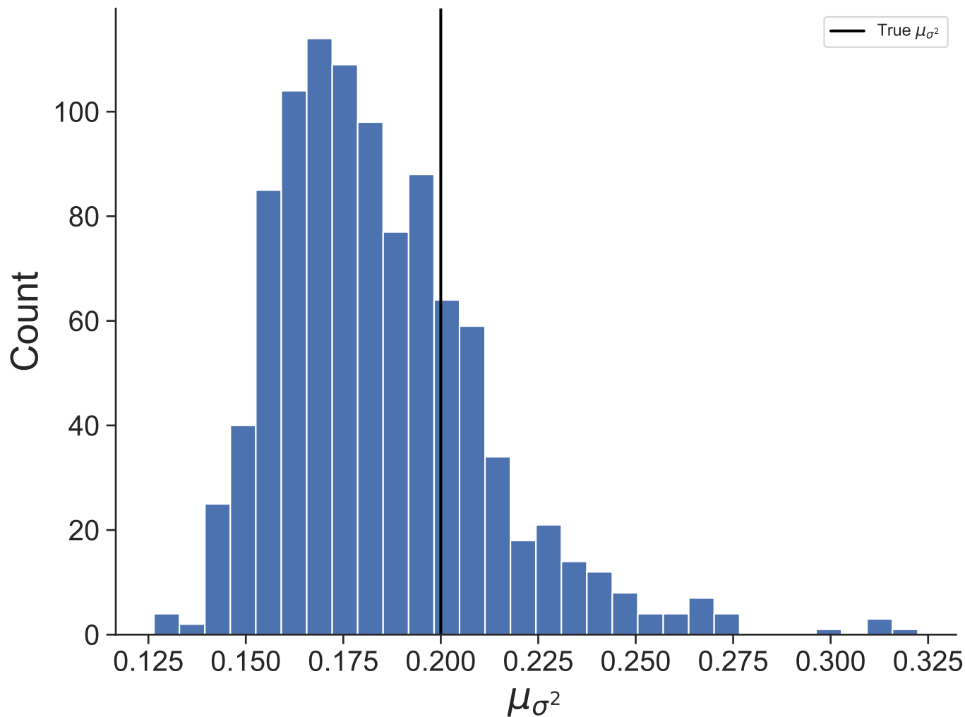
Dataset 45
