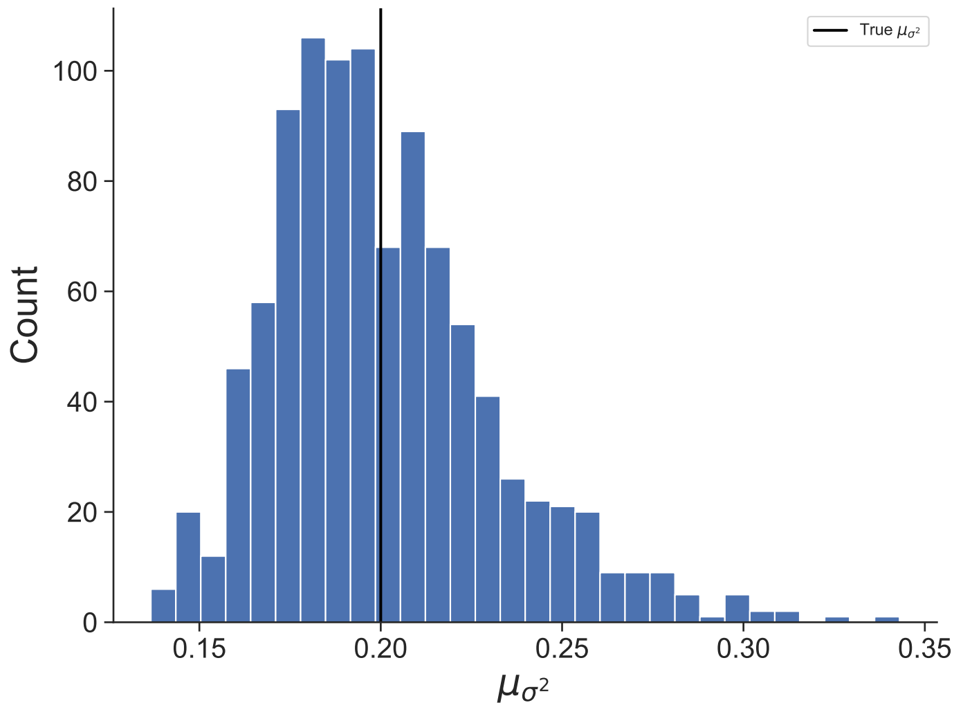
Dataset 23
