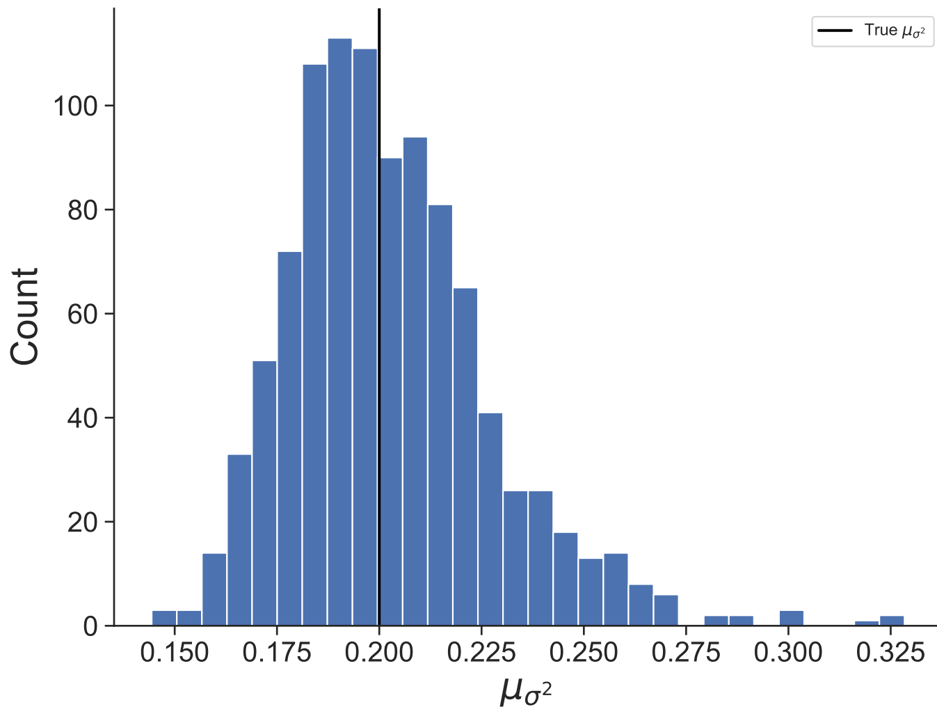
Dataset 5
