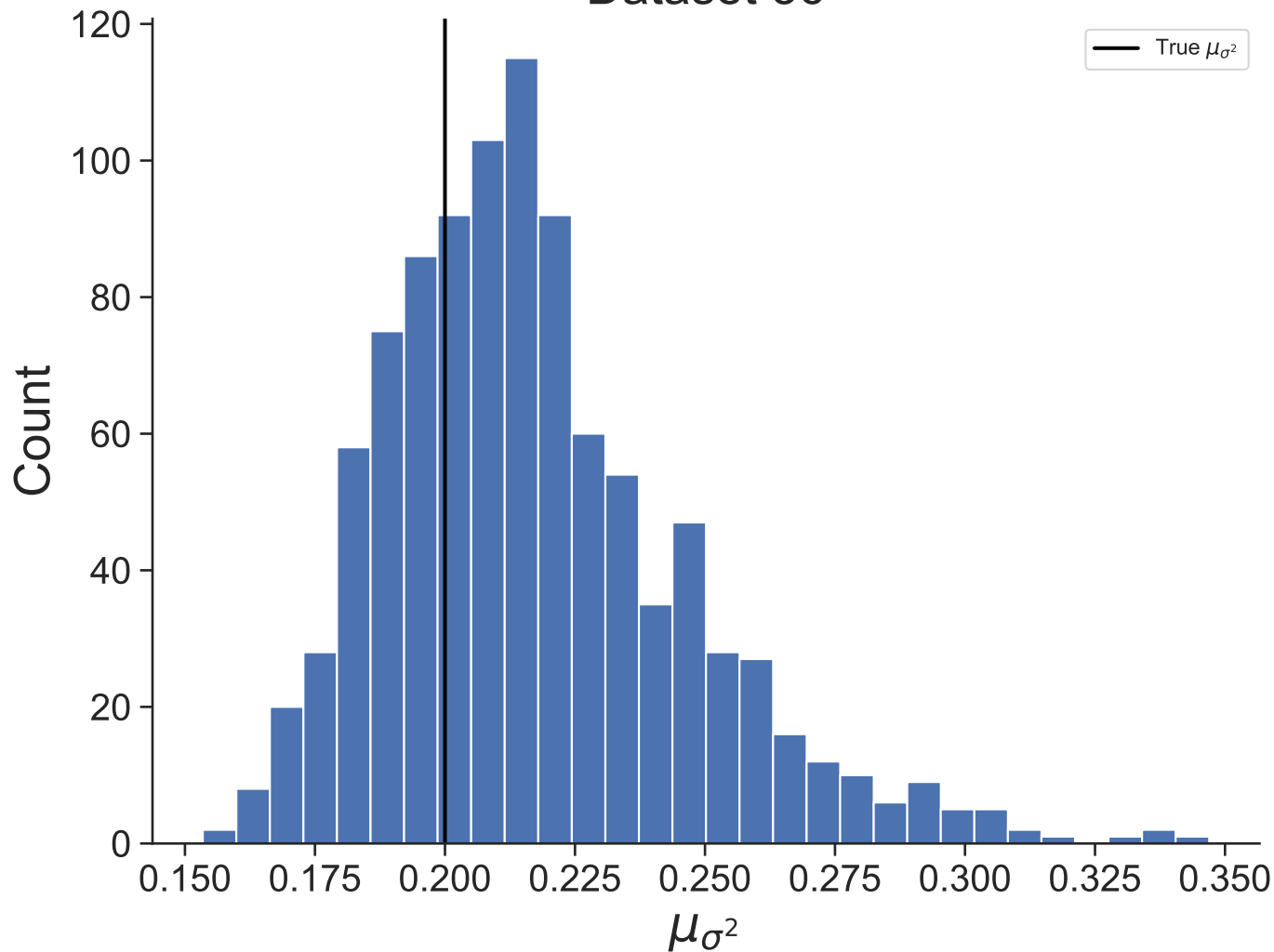
Dataset 36
