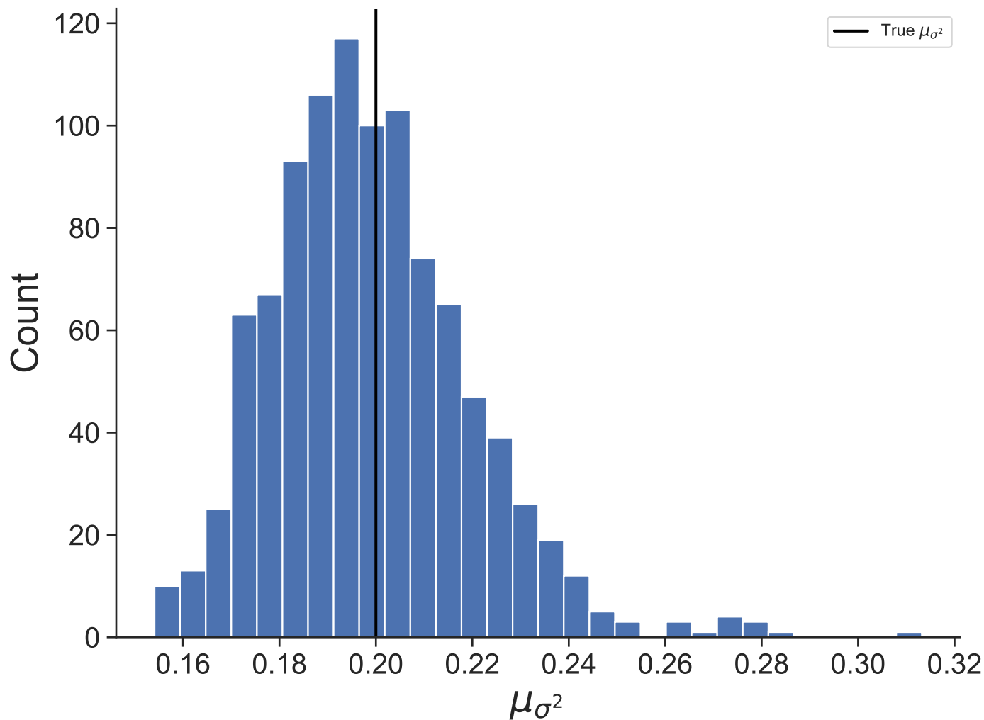
Dataset 13
