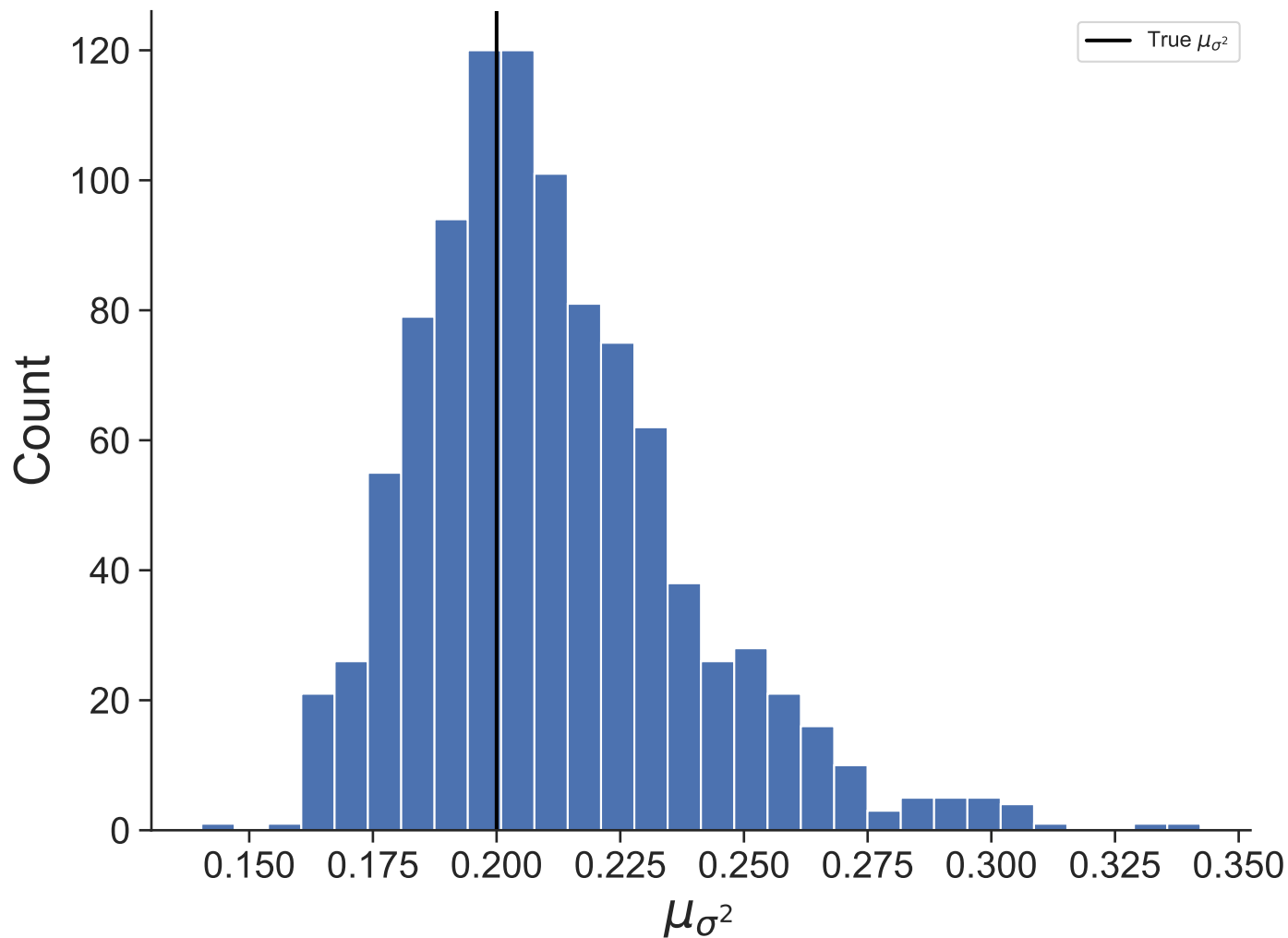
Dataset 4
