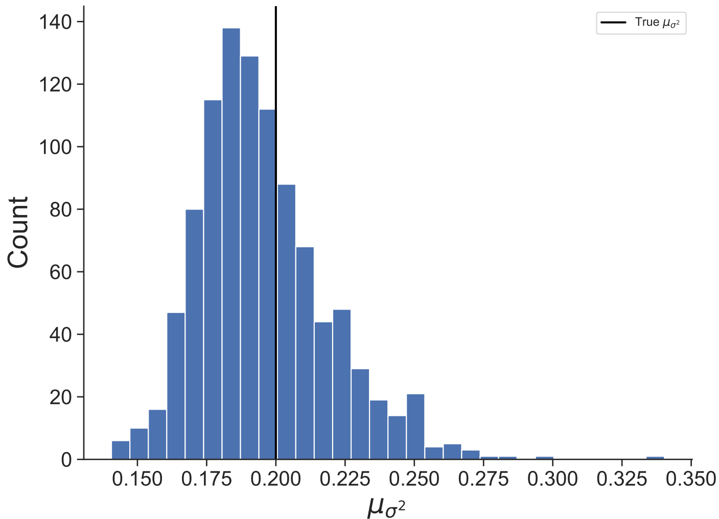
Dataset 17
