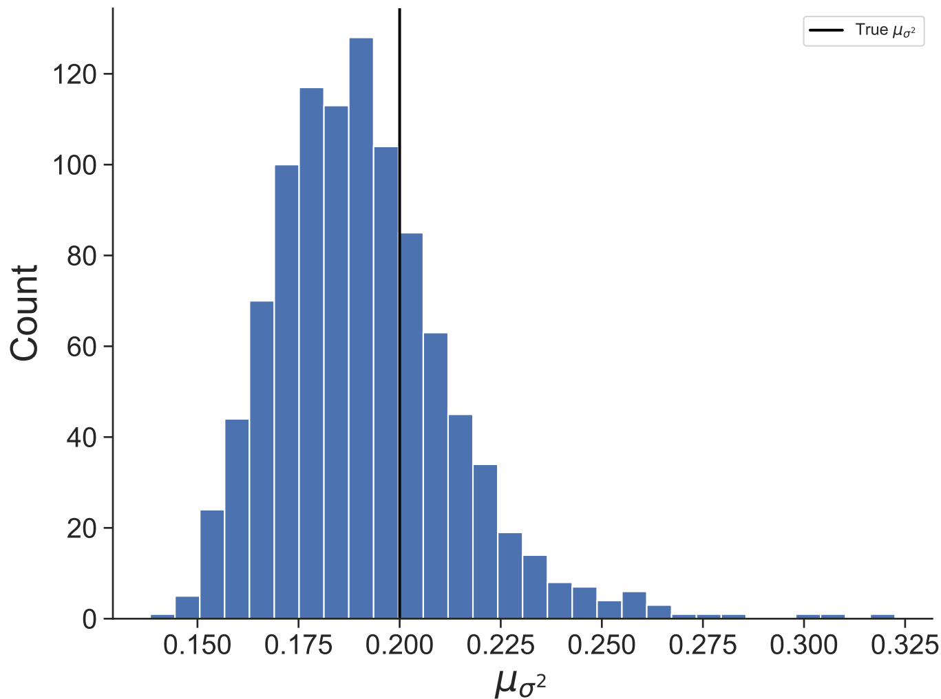
Dataset 14
