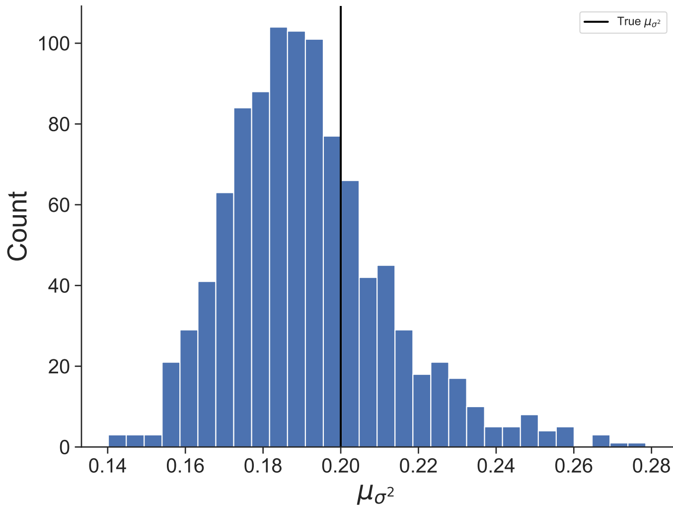
Dataset 42
