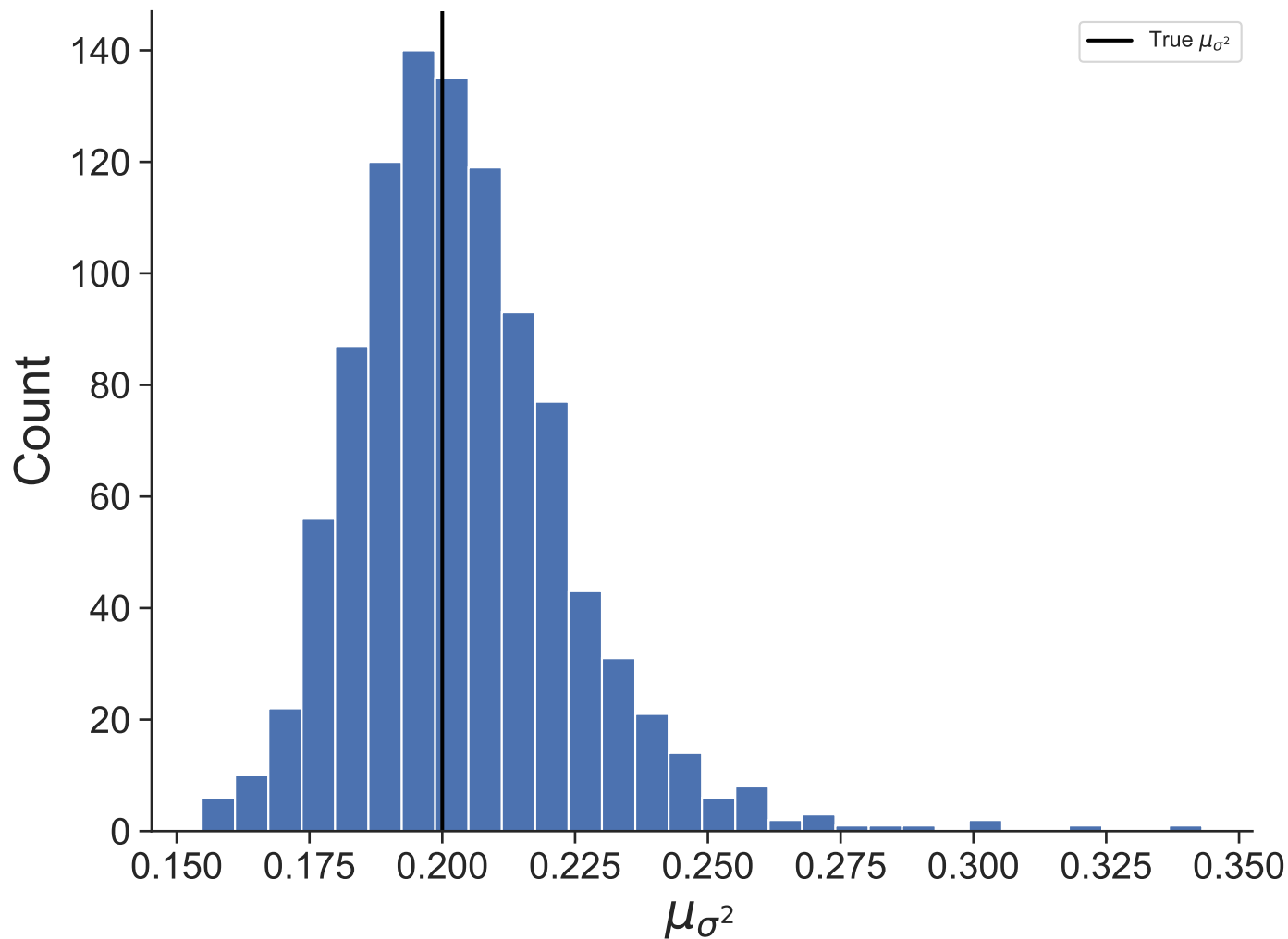
Dataset 10
